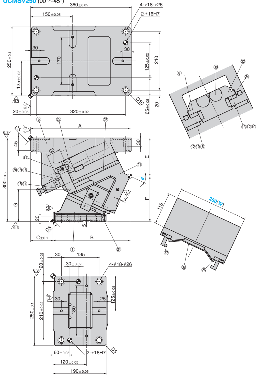
UCMSV250 (00°~45°)
